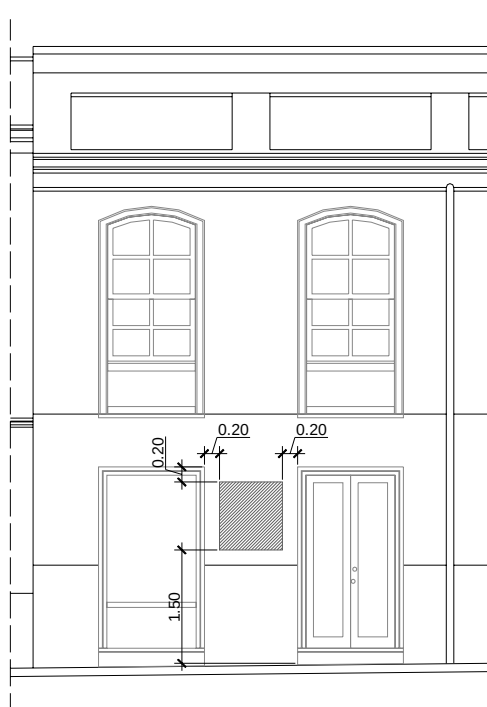
Tipo 1. Área de movimiento del rótulo en los paños de fachada entre vanos
