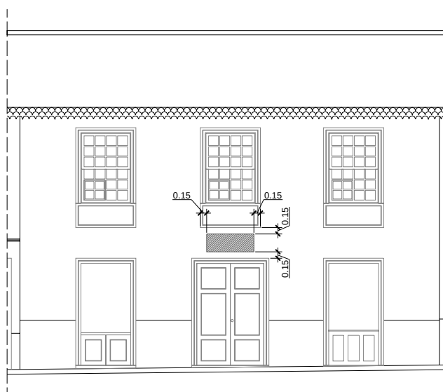
Tipo 1. Área de movimiento del rótulo en los paños de fachada entre vanos
